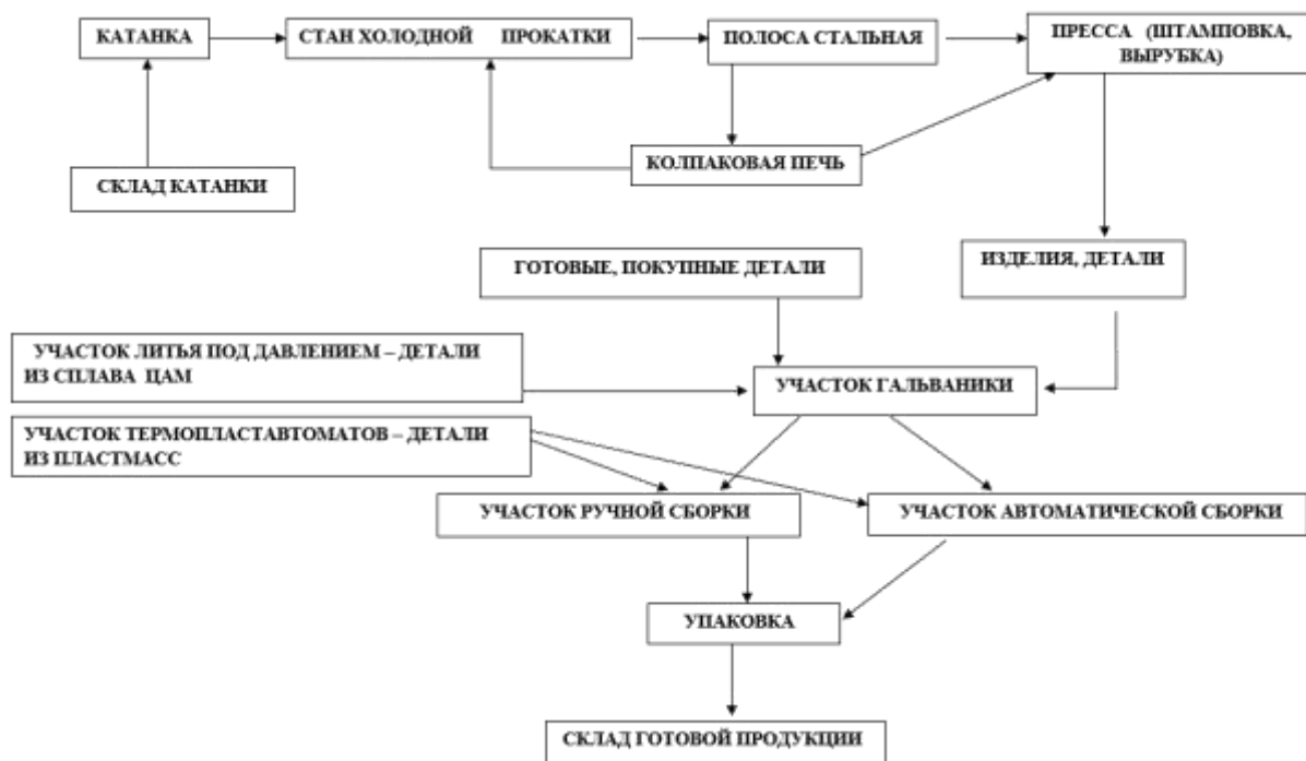
Рис. 3.3. Схема технологического процесса производства фурнитуры
