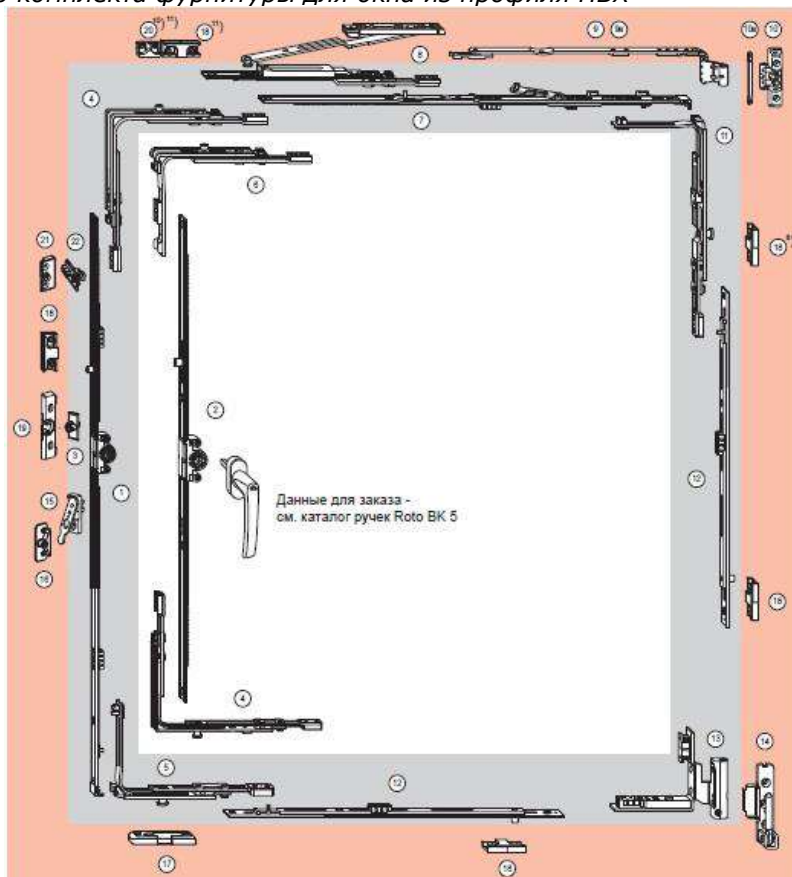
Рис. 3.2. Пример комплекта фурнитуры для окна из профиля ПВХ
